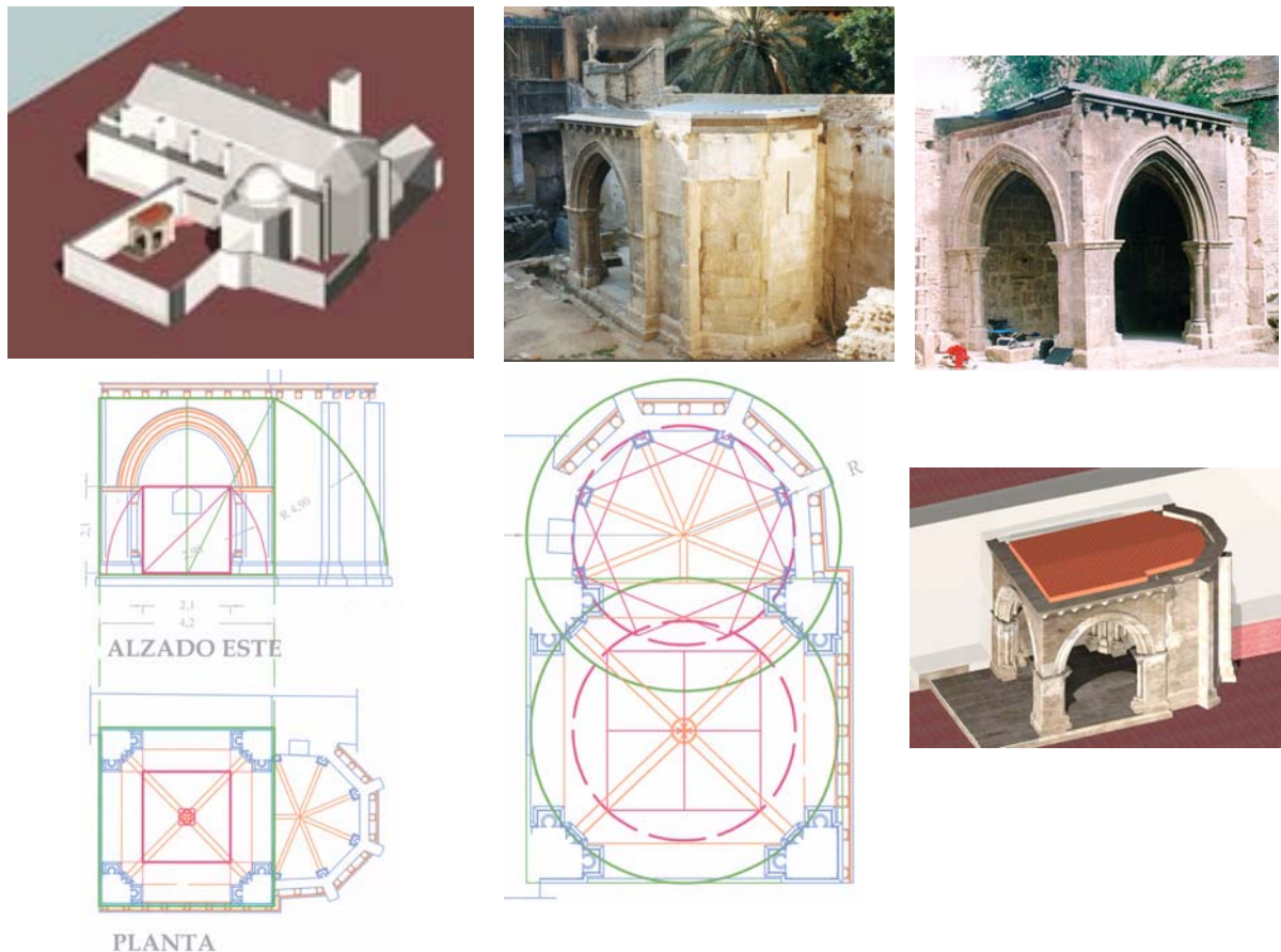
Fig. 3 Resultados del campo de trabajo realizado en 2001 por alumnos de la ETSGE para el levantamiento y estudio geométrico de la Capilla Funeraria del Cementerio medieval de la iglesia de San Juan del Hospital de Valencia
