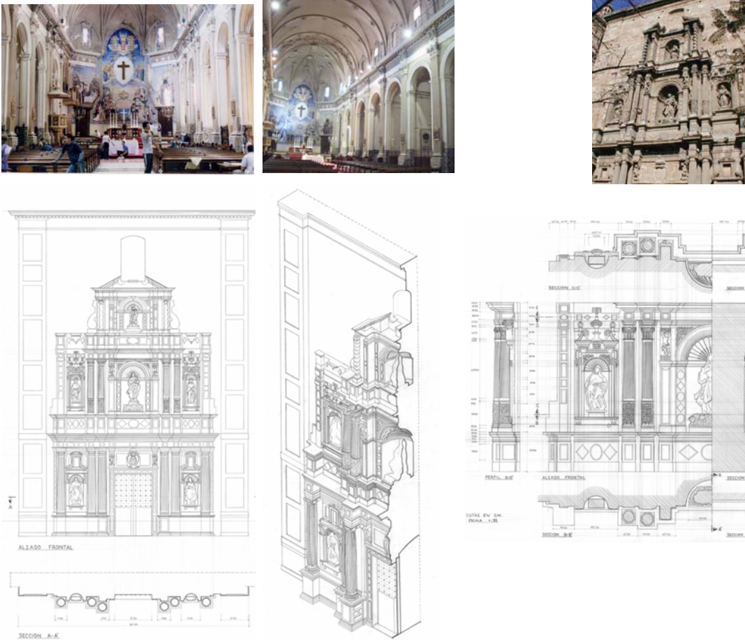
Fig. 4 Resultados del campo de trabajo realizado por alumnos de primer curso de la ETSGE en 2001 para el levantamiento de la iglesia de la Santísima Cruz de Valencia
