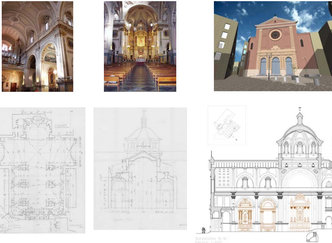
Fig.1 Resultados del Campo de Trabajo realizado con alumnos de la ETSGE en 2002 para el levantamiento de planos de la iglesia de la Compañía de Jesús de Valencia
