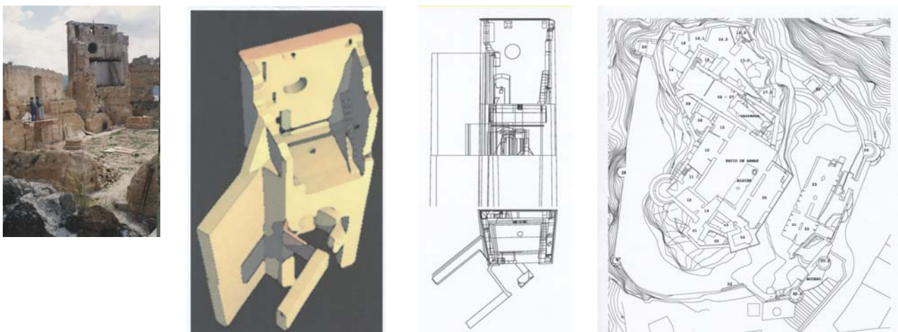
Fig. 2 Resultados del campo de Trabajo realizado en 1999 con alumnos de ETSGE para el levantamiento y estudio de los materiales del Castillo de Cofrentes
